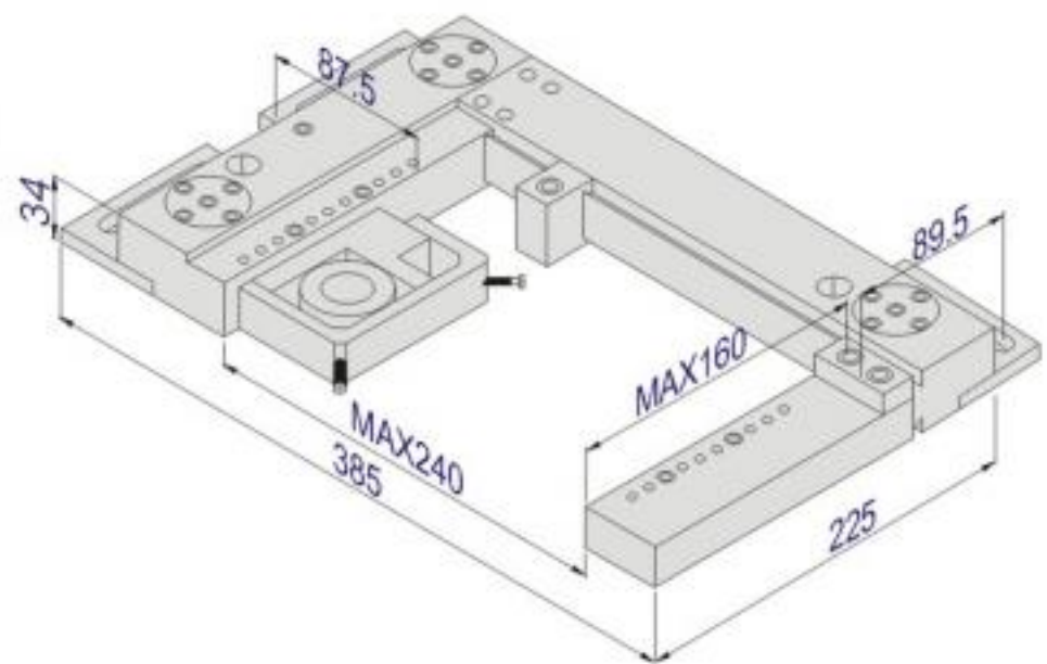
裝夾位置關係圖
