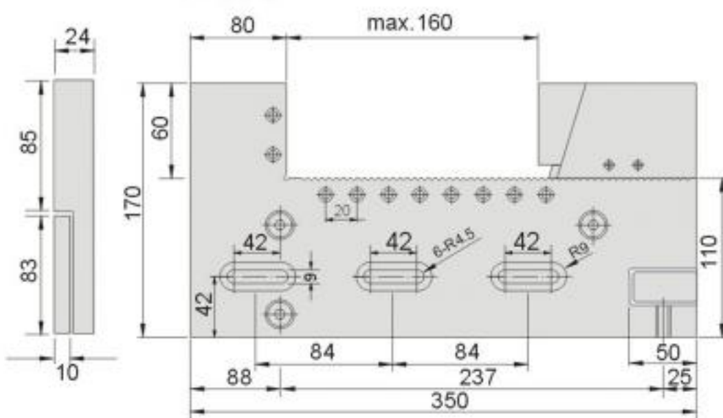
WPV320尺寸圖
