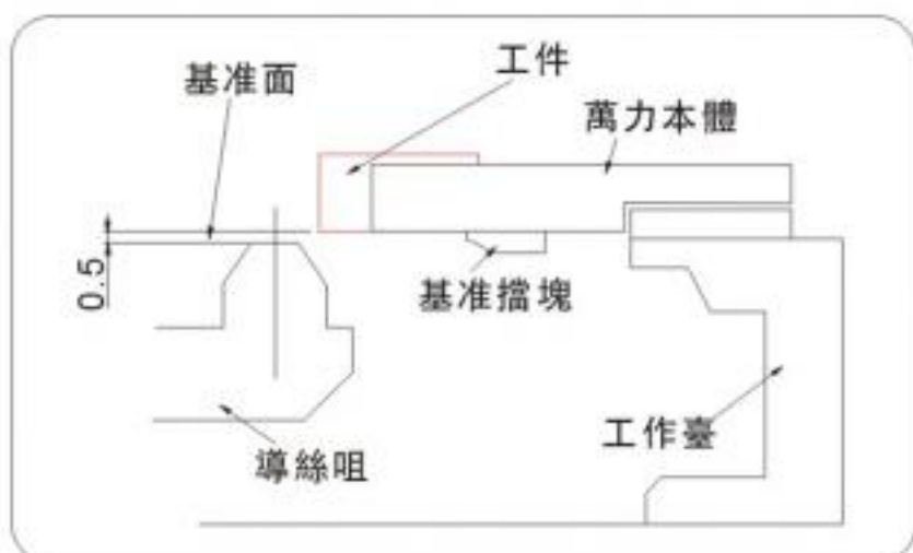
裝夾位置關係圖
