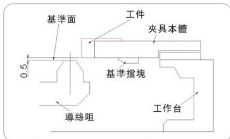
WPV320尺寸圖
