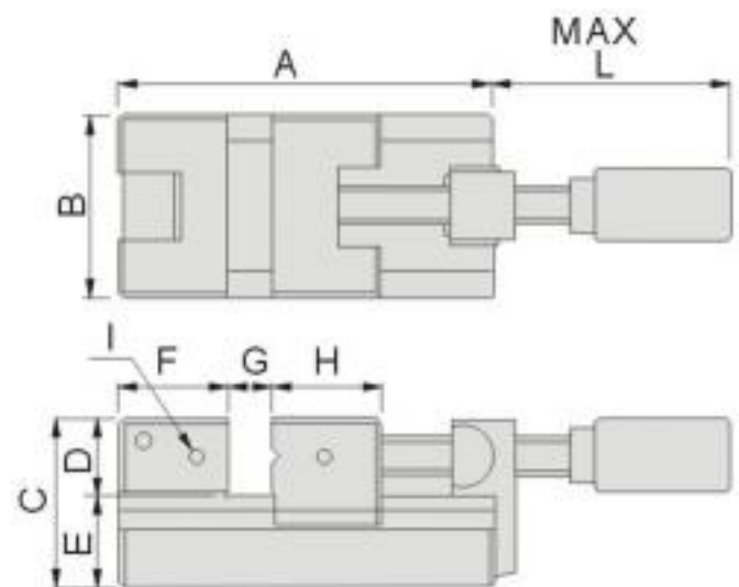
HU60/70示意圖
