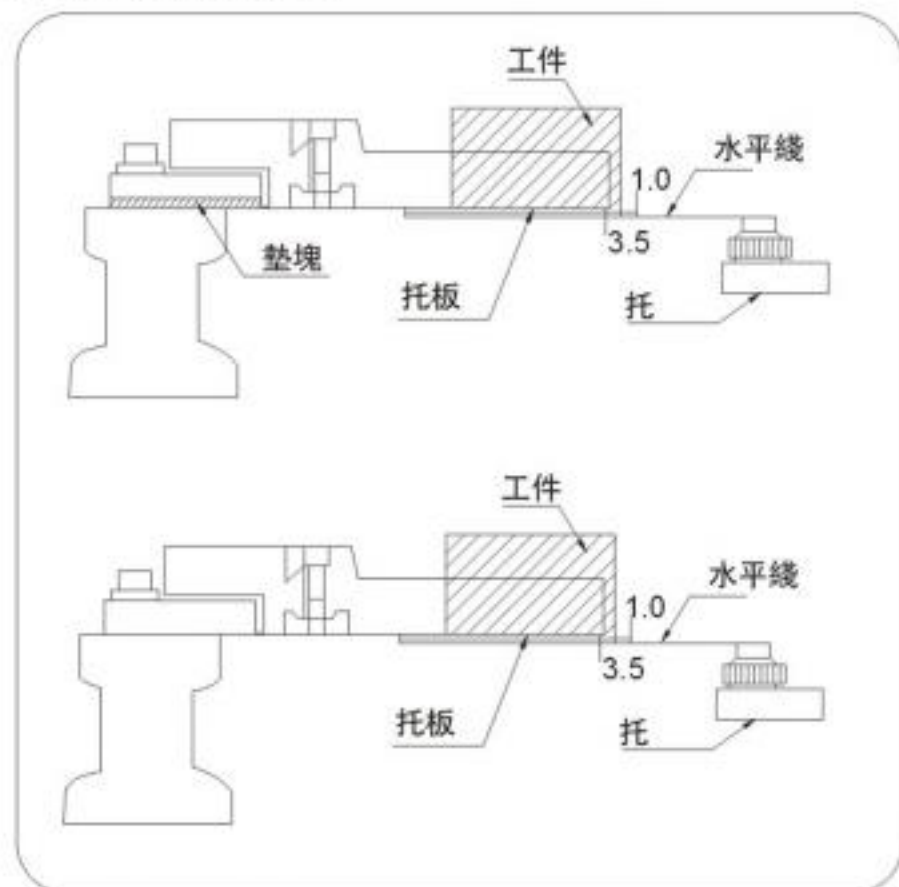
裝夾位置關係圖
