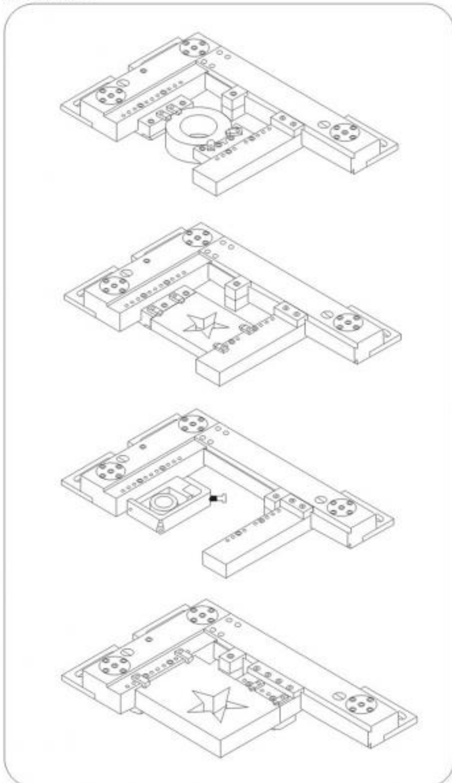
裝夾位置關係圖
