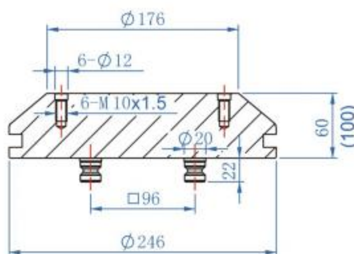
剖面圖 A-A
